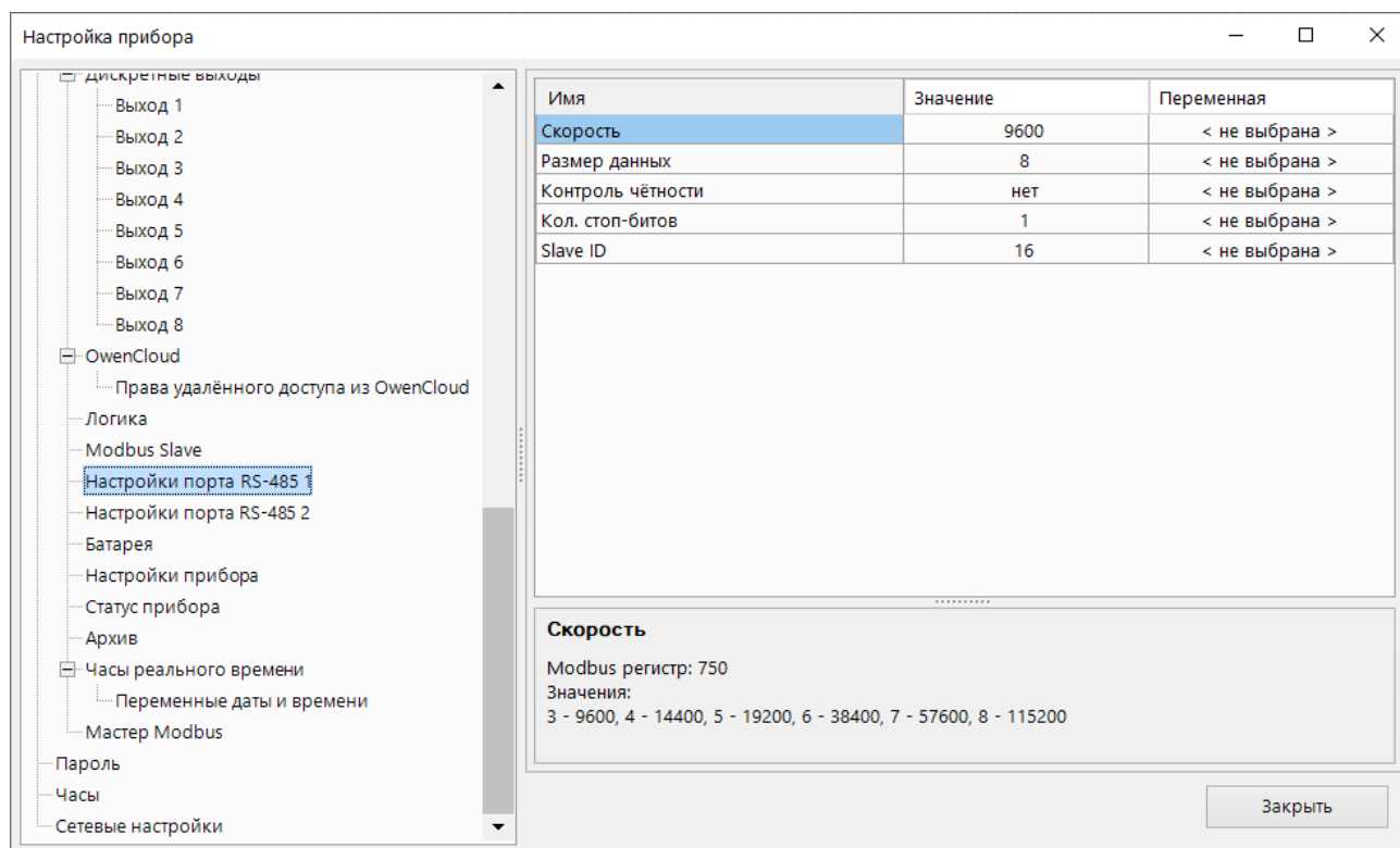
Рисунок 4.17 – Настройки параметров RS-485
